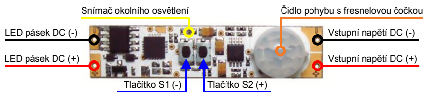
Obr.1 - Zapojení vývodů a umístění ovládacích prvků
